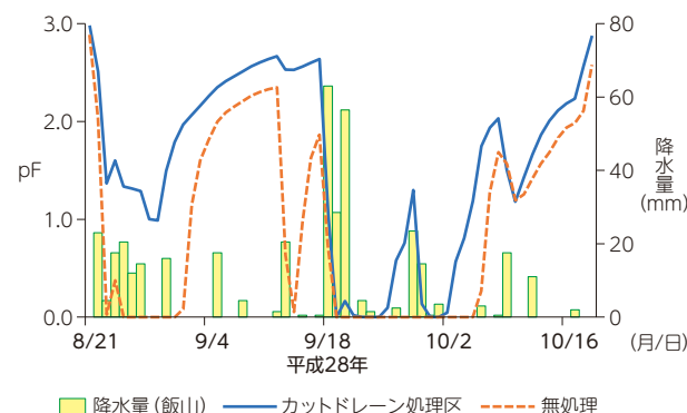
図3 カットドレーン処理が土壌pFに及ぼす影響（平成28年、野菜花き試験場）
