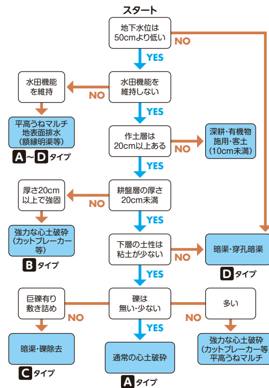
図2 水田転換畑のブロッコリー栽培における排水対策フロー図(2021年、野菜花き試験場)
