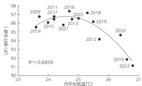
図1 8月の月平均気温と長野県の一等米比率 気温データはアメダス観測地点穂高を使用。(2009～2023年)
